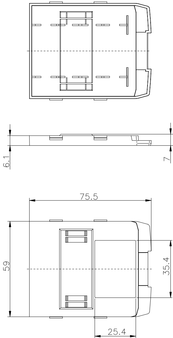
Akkufachdeckel/ lid
