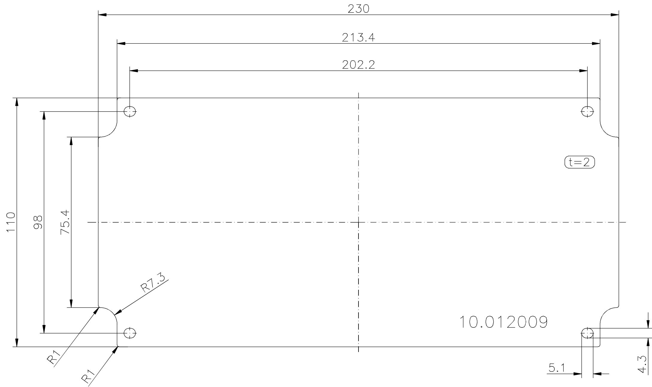
Montageplatte Bestell-Nr.: 10.012009
